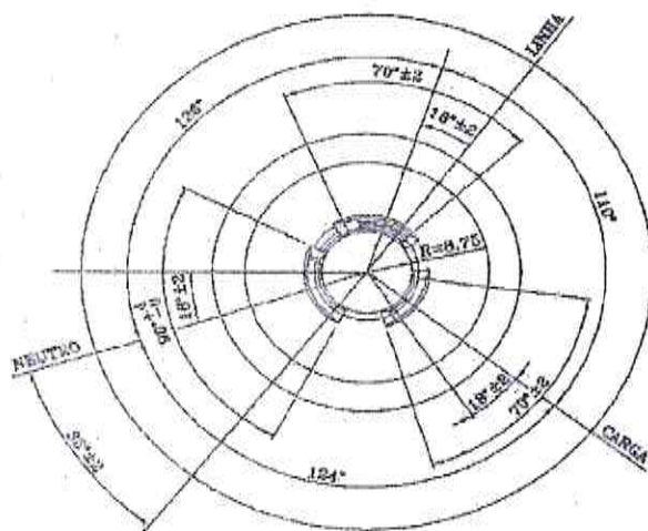
VISTA INFERIOR
