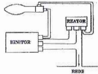
DETALHE 1
