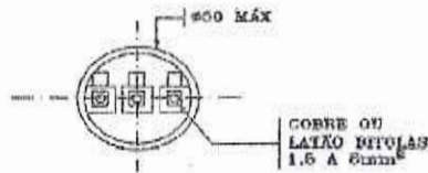
VISTA INFERIOR
